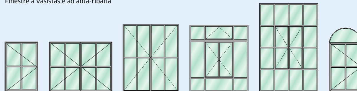
Finestre a vasistas e ad anta-ribalta
